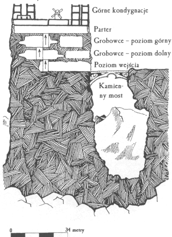
PRZEKRÓJ POPRZECZNY ORLEGO GNIAZDA
