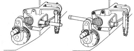
Буксирная серьга
