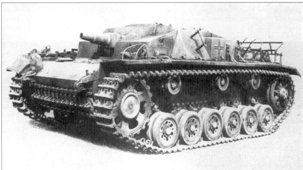
Установка Sturmgeschütz Ausf. D (Fgst.Nr. 90683) была одной из трех штурмовых орудий, переброшенных в Северную Африку в составе зондеркоманды 288. Машина «тропикализирована» путем установки дополнительных воздушных фильтров и увеличения притока воздуха в моторное отделение через дополнительные отверстия в крышках люков крыши задней части корпуса. Обратите внимание на смятое бронирование смотровой щели механика-водителя - след попадания противотанкового снаряда. В кормовой части корпуса видна сварная конструкция для крепления канистр с дополнительным запасом воды и топлива.
