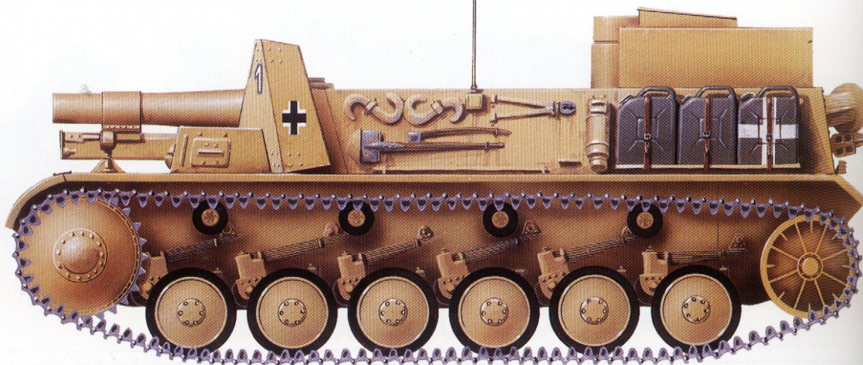
15cm s.I.G.33 B Sfl., s.I.G.Kp.(mot.S) 707 or 708, Libya, 1942
