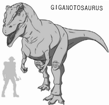
GIGANOTOSAURUS
