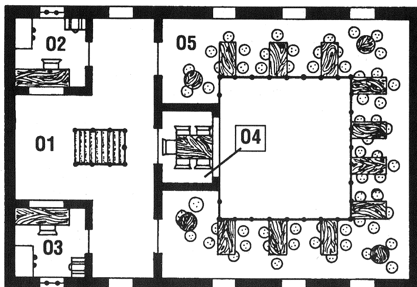
Obergeschoß
