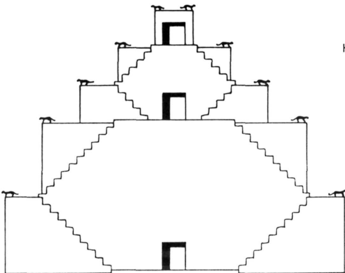
Ansicht
