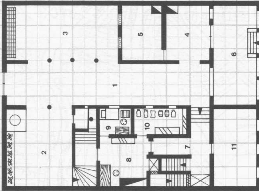
Erdgeschoß (E)
