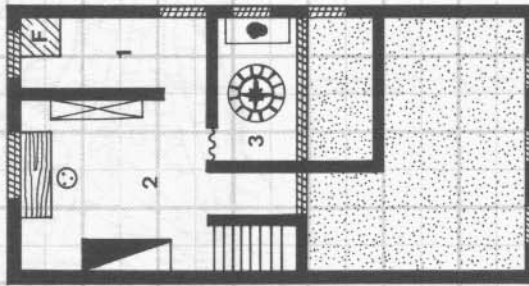
Untergeschoß (U)
