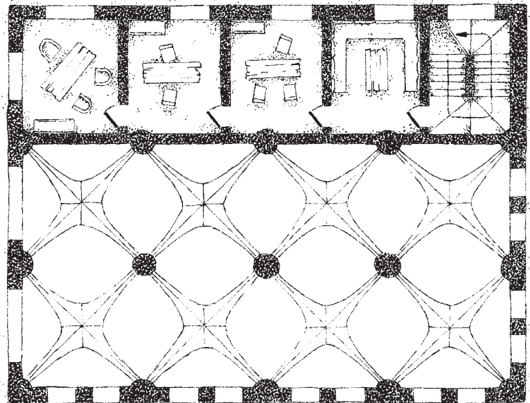
Zwischengeschoss
