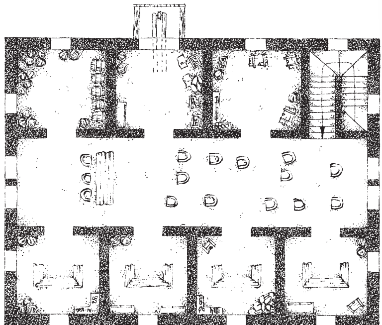
Obergeschoss
