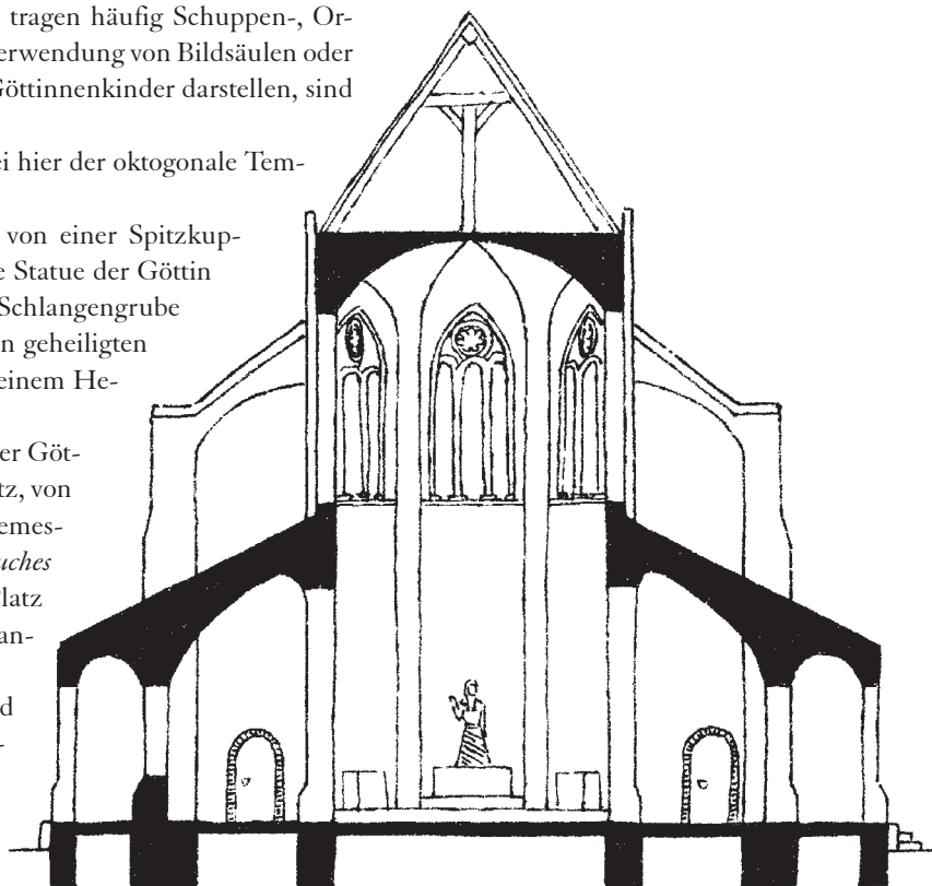
Querschnitt
