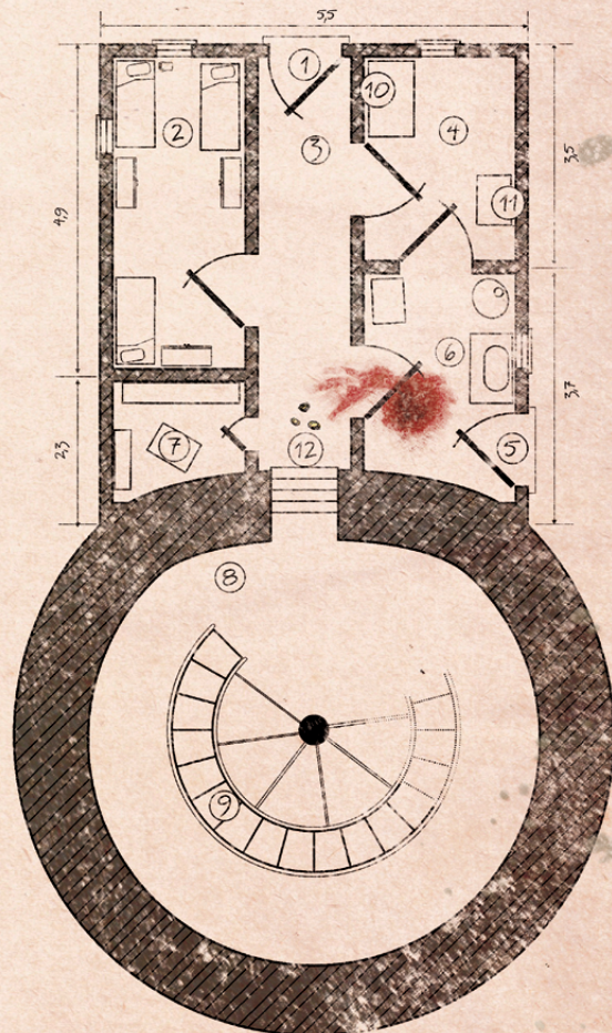
PLANTA BAIXA
