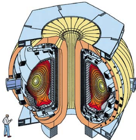
Anlagenschema eines Tokamak
